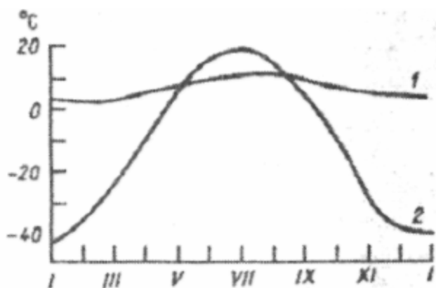
Рис. 3.2. Годовой ход температуры воздуха на широте 62^{\circ} с.ш. в Торсхавне и Якутске: 1 – Торсхавна; 2 – Якутск
