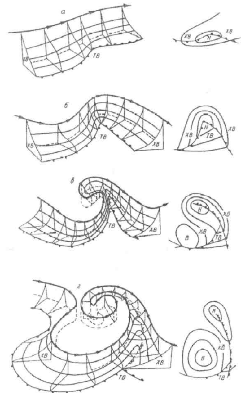
Рис. 7.7. Формирование циклона
