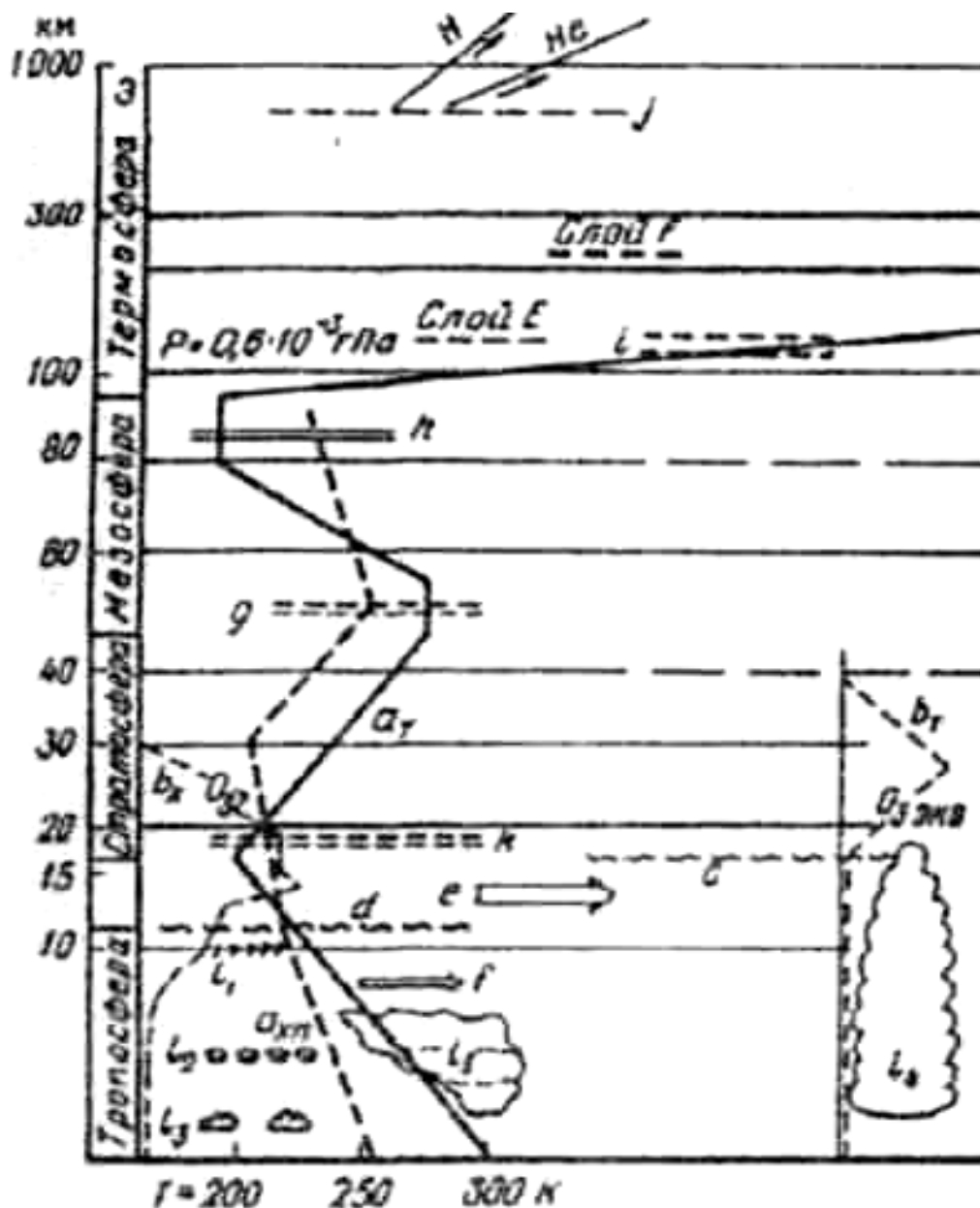
Рис. 1.1. Строение атмосферы: a – распределение температуры ( a_m – в тропиках, a_{хл} – в холодной полярной зоне); b_m и b_n – распределение озона в тропической и полярной зонах; c – тропопауза тропическая; d – тропопауза полярная; e – струйное течение субтропическое; f – струйное течение полярное; g – стратопauses; h – мезопauses; i – турбопауза; j – уровень диссипации – ускользания атомов H и He; k – слой атмосферного аэрозоля; l_1, l_2, l_3, l_4, l_5 – тропосферные облака: перистые, высококучевые, кучевые, кучево-дождевые, фронтальные; \varepsilon – экзосфера
