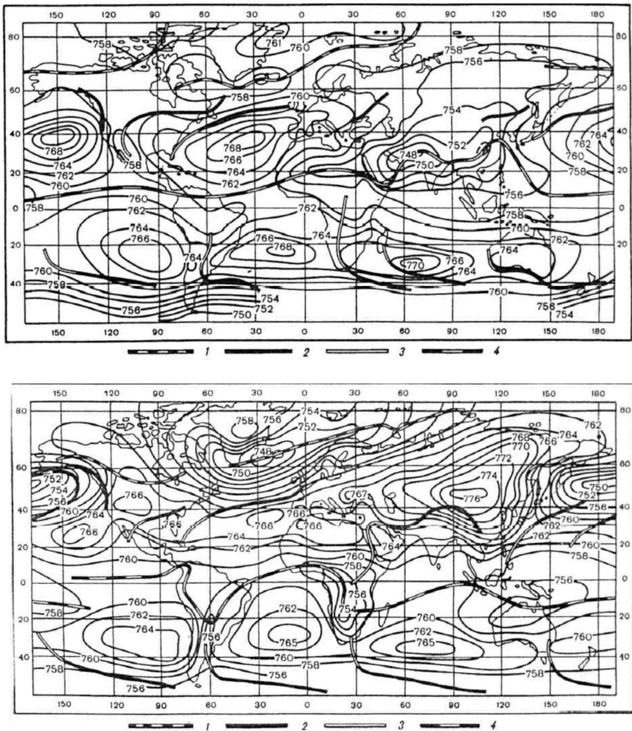
Рис. 7.4, 7.5. Климатологические фронты в июле и январе
