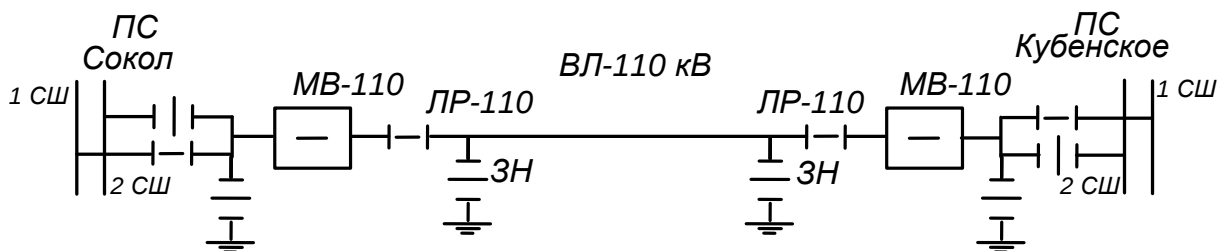
Рис. 15. Схема ВЛ 110 кВ двустороннего питания
