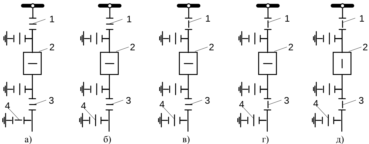
Рис. 14. Очередность операций по включению коммутационных аппаратов линейной ячейки 10 кВ: а) исходная схема; б) отключены заземляющие ножи линейного разъединителя в сторону линии (проверяется отключенное положение выключателя); в) включен шинный разъединитель; г) включен линейный разъединитель; д) включен выключатель
