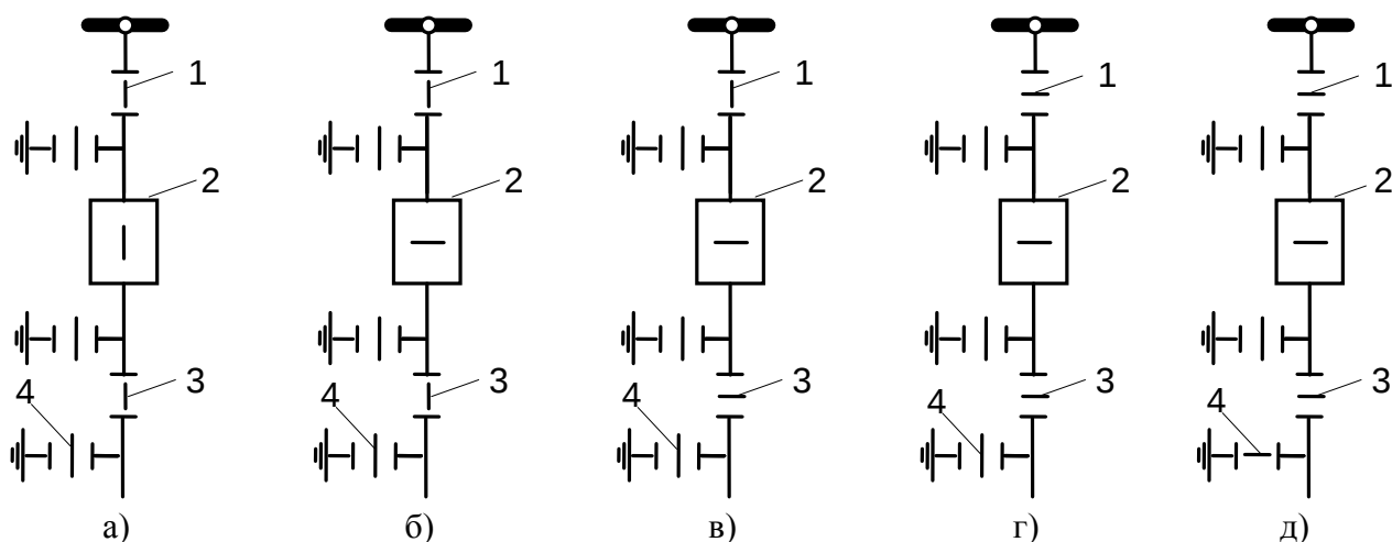
Рис. 13. Очередность операций по отключению коммутационных аппаратов линейной ячейки 10 кВ: а) исходная схема; б) отключен выключатель; в) отключен линейный разъединитель; г) отключен шинный разъединитель; д) включены заземляющие ножи линейного разъединителя в сторону линии
