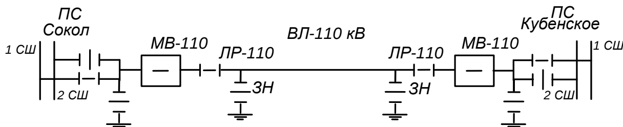
Рис. 19 Схема линии с двухсторонним питанием
