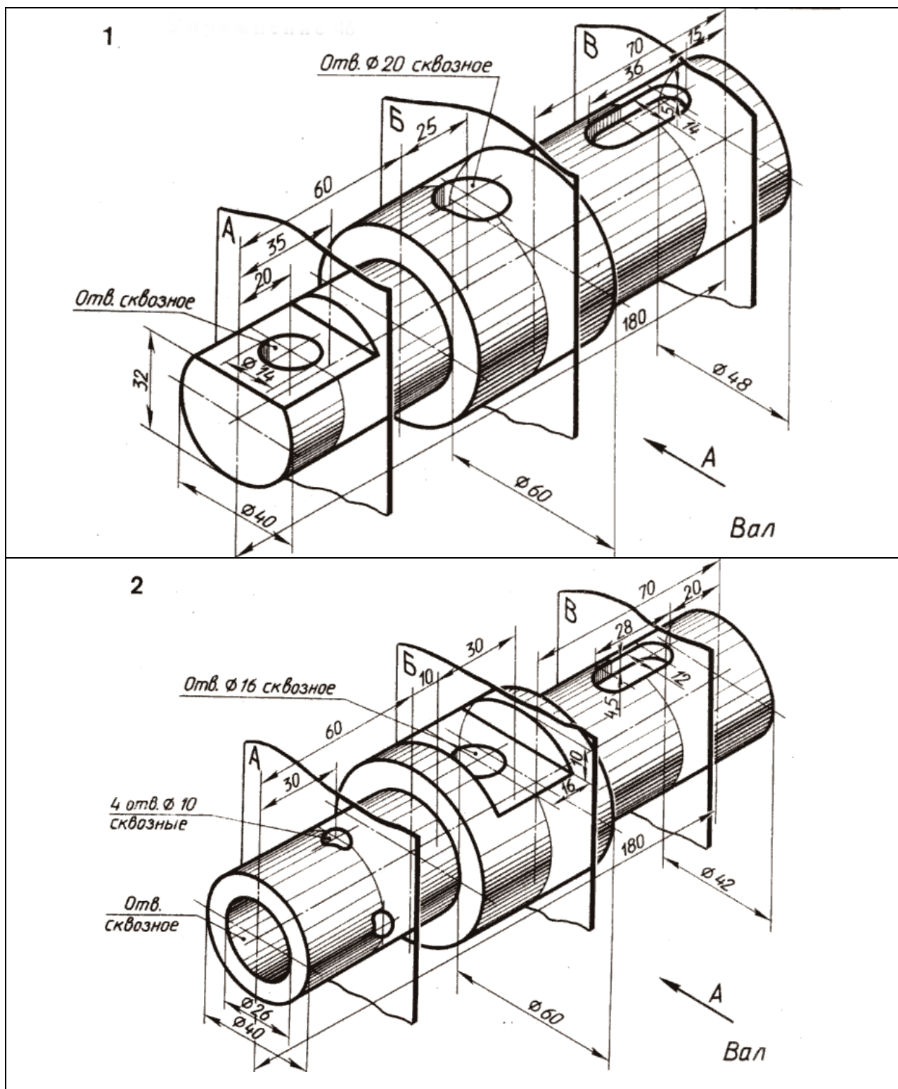
Рисунок 7.3- Задание по теме «Сечения»
