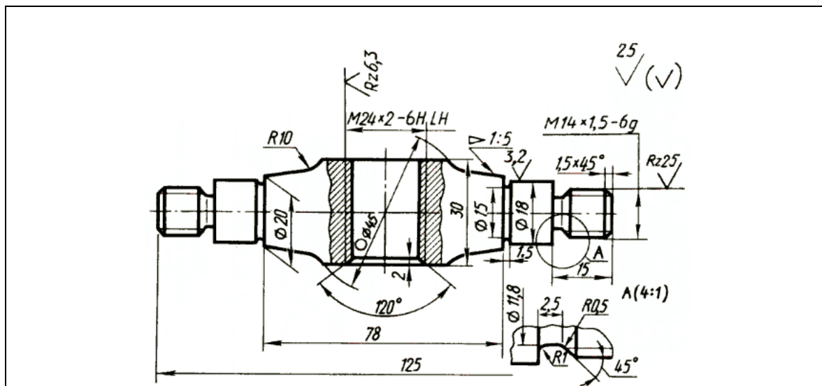
Рисунок 8.11 – Пример выполнения рабочего чертежа детали с выносным элементом – наружной проточкой
