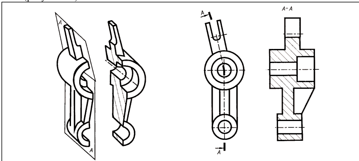
Рисунок 6.2 – Ломаный разрез
