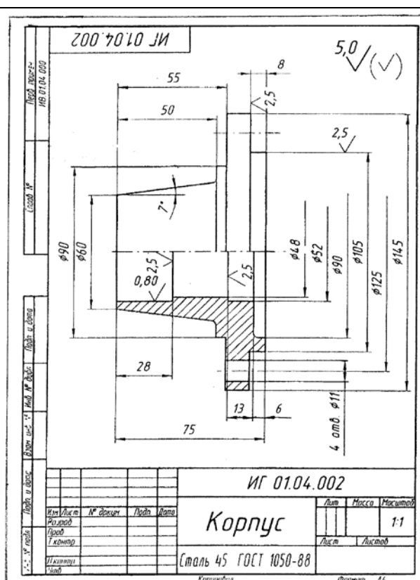
Рисунок 8.10 - Пример выполнения рабочего чертежа детали вращения
