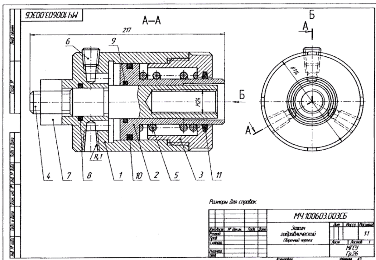
Рисунок 8.8 - Чертеж сборочной единицы
