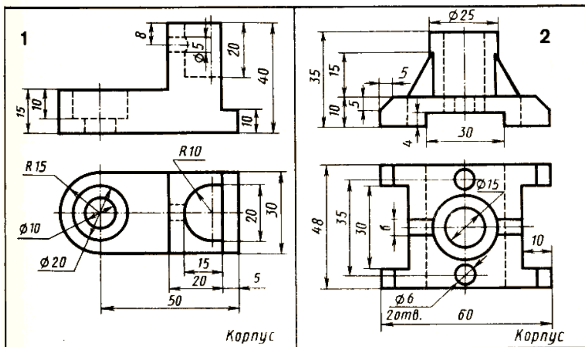
Рисунок 5.2- Задание по теме «Простые разрезы»
