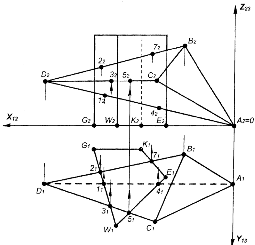
Рисунок 2.4 – Построение точек пересечения ребер пирамиды с призмой
