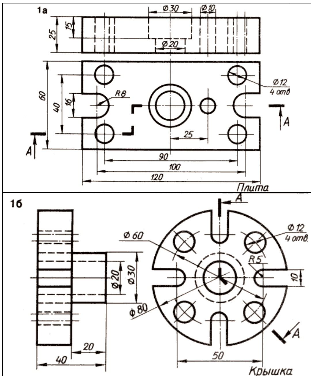
Рисунок 6.3 – Задание по теме «Сложные разрезы»
