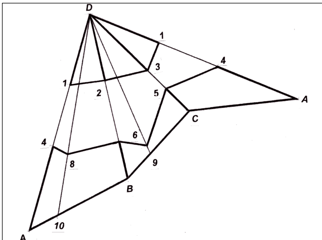
Рисунок 3.6 – Развертка боковой поверхности пирамиды
