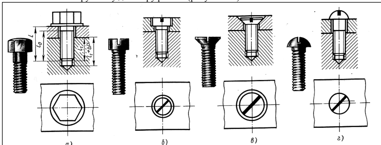
Рисунок 8.3 - а) болтовое соединение двух деталей, б) соединение винтом с цилиндрической потайной головкой, в) соединение винтом с конической потайной головкой, г) - соединение винтом с полукруглой головкой
