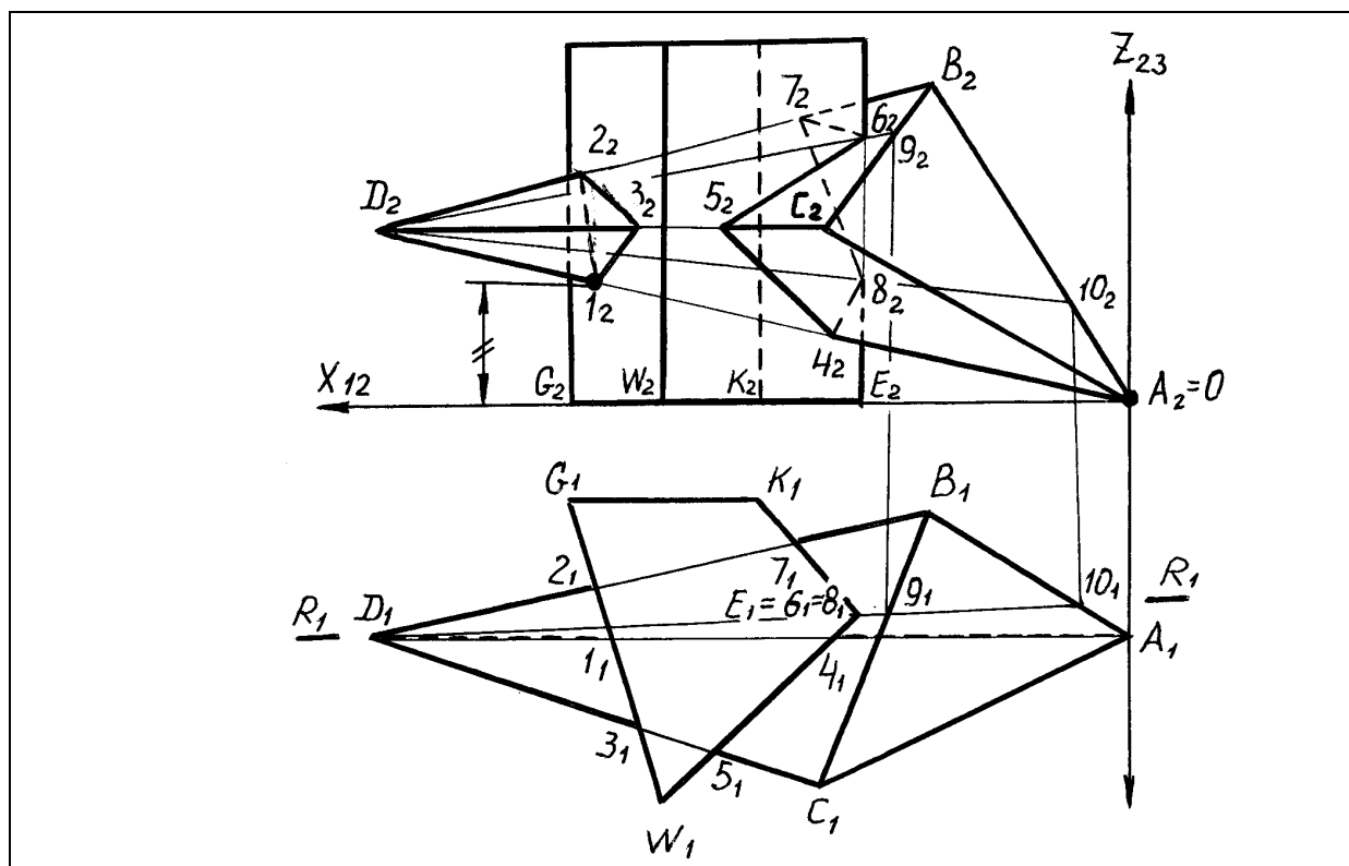
Рисунок 3.1 – Пирамида и призма с линиями пересечений
