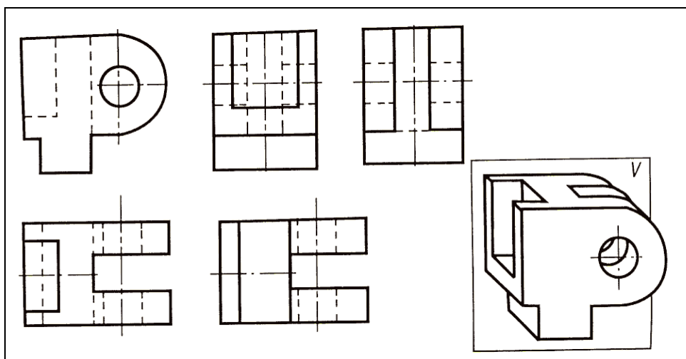
Рисунок 4.5 – Основные виды вне проекционной связи
