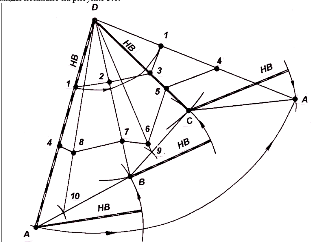
Рисунок 3.5 – Схема построения развертки боковой поверхности пирамиды
