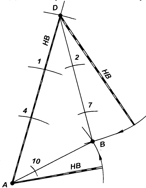
Рисунок 3.4 – Построение грани пирамиды по трем известным сторонам
