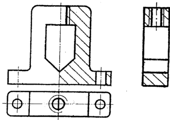
Рисунок 5.1- Пример выполнения простых разрезов
