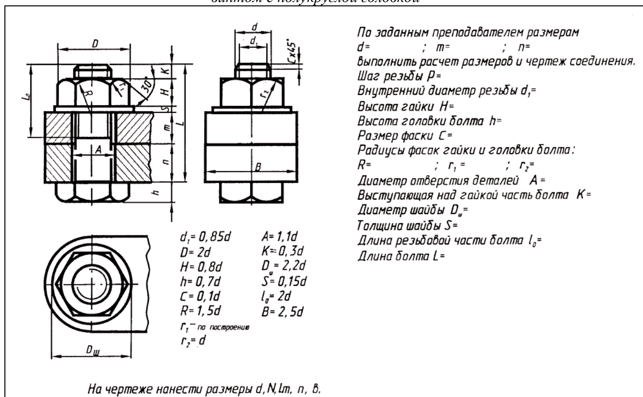
Рисунок 8.4 – Схема выполнения изображения соединения деталей болтом
