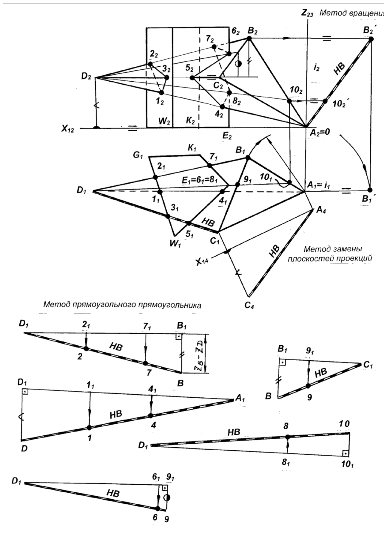
Рисунок 3.3 – Определение натуральных величин ребер пирамиды
