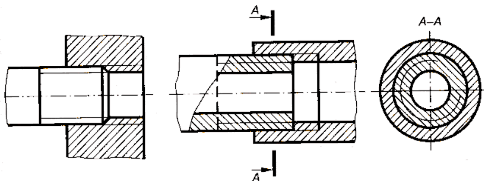
Рисунок 8.2-Изображение резьбы не зависит от типа резьбы
