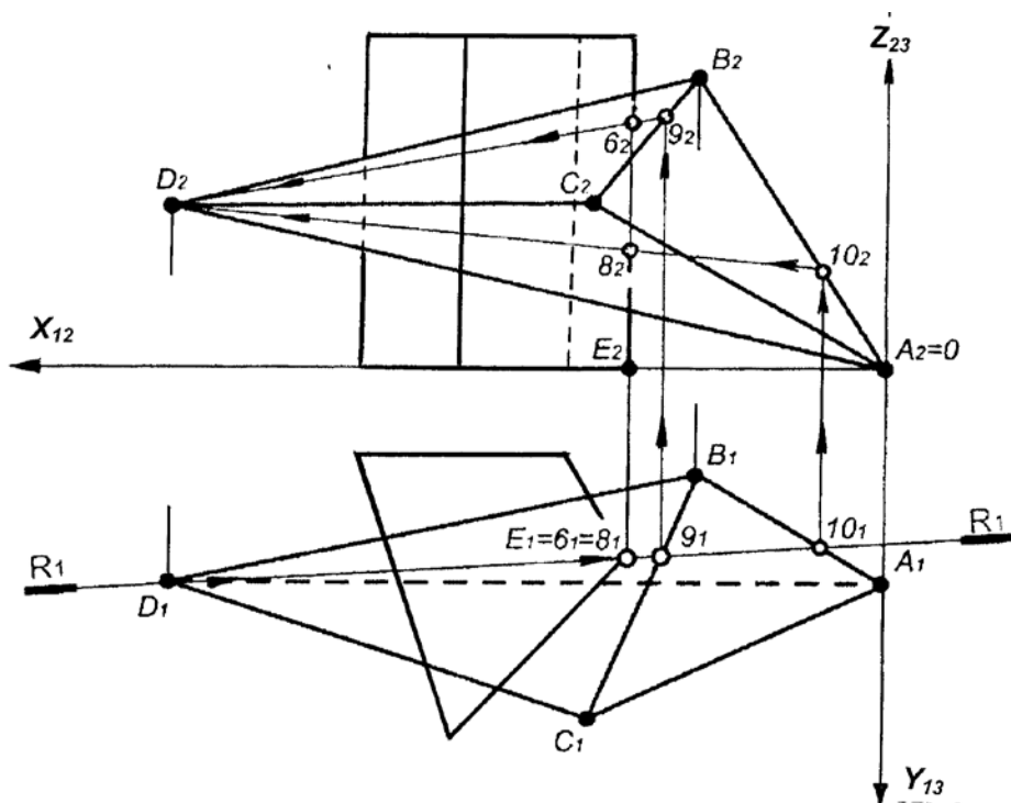
Рисунок 2.5 – Построение точек пересечения ребра призмы E с гранями пирамиды
