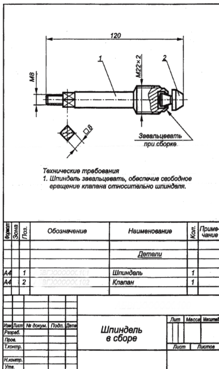
Рисунок 8.7 – Пример сборочного чертежа на формате А4
