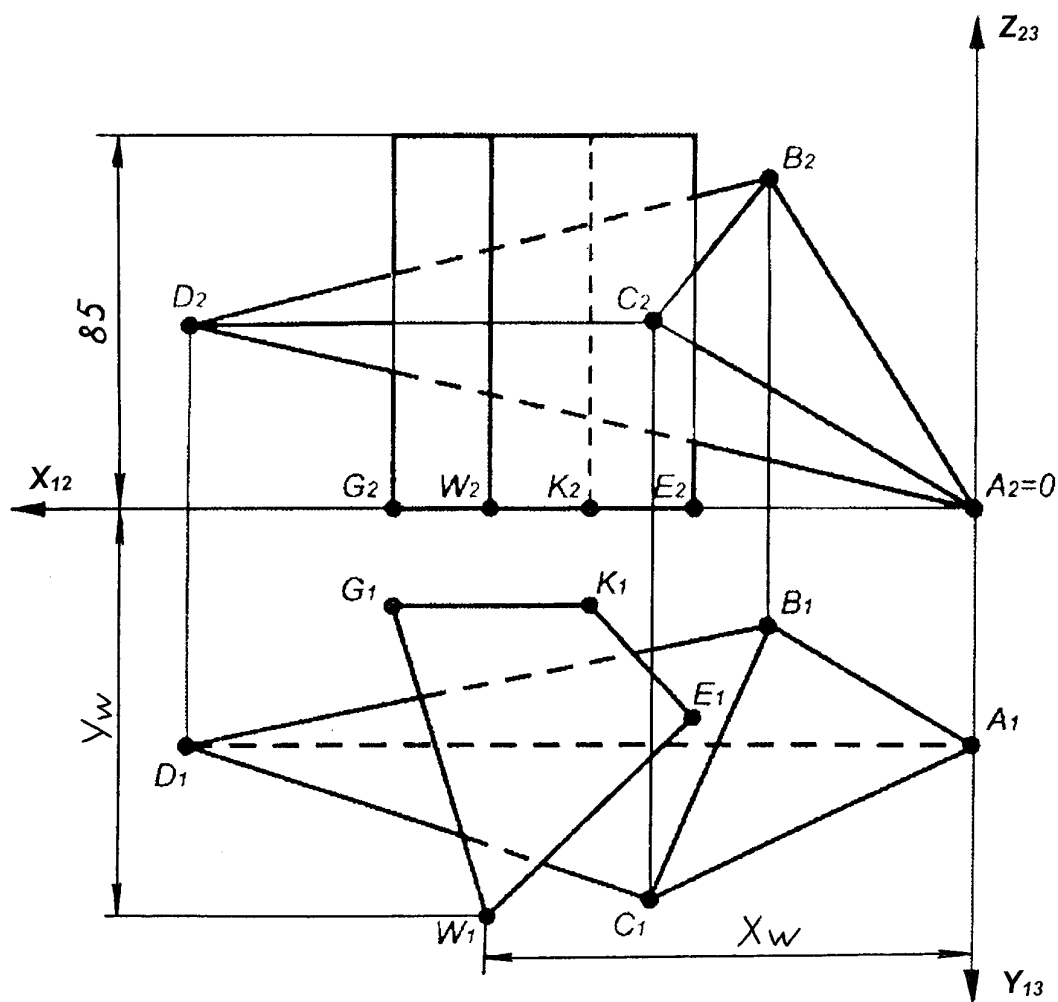
Рисунок 2.3 – Построение проекций призмы с основанием GWTK
