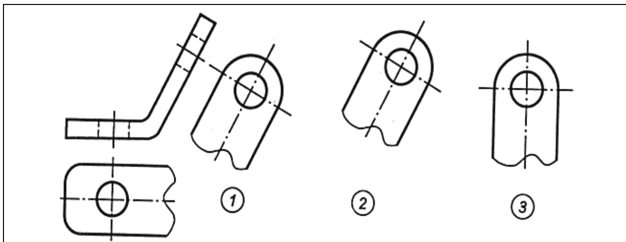
Рисунок 4.4 – Дополнительные виды
