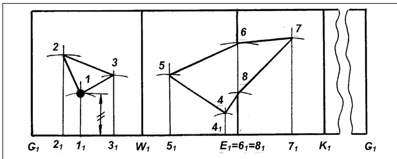
Рисунок 3.2 – Развертка боковой поверхности призмы
