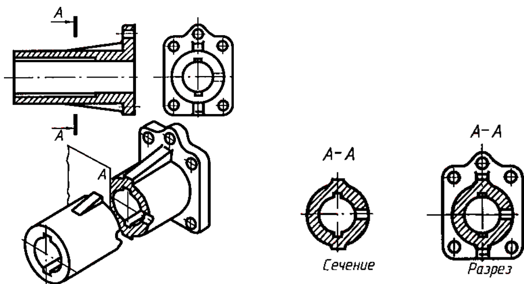
Рисунок 7.1-Различие между сечением и разрезом
