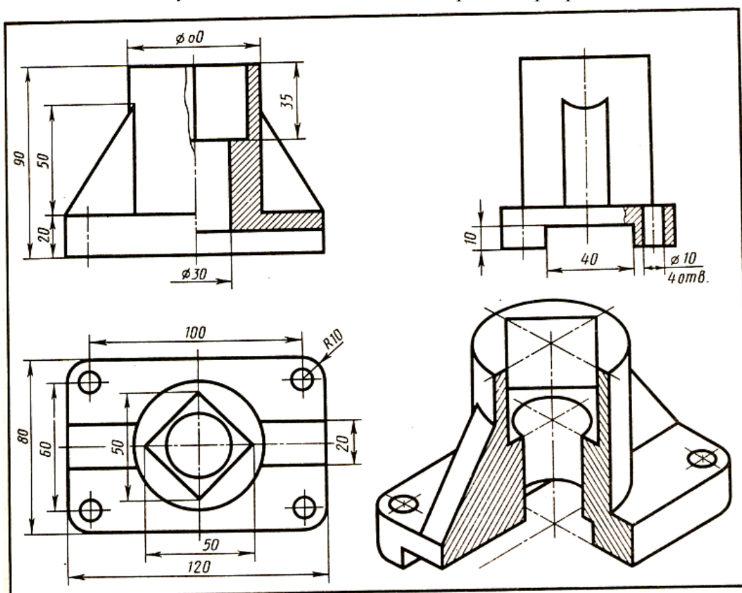
Рисунок 5.3 –Пример выполнения листа 3
