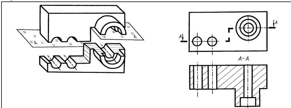
Рисунок 6.1 – Ступенчатый разрез
