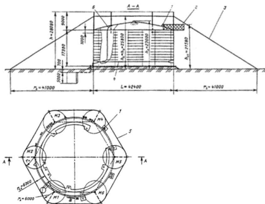
Рис. 7. Молниезащита металлического резервуара вместимостью 20 тыс. м 3 со сферической крышей и понтоном:
