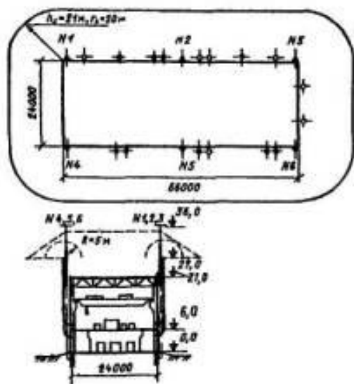
Рис. 5. План цеха компрессии азотоводородной смеси (относится к взрывоопасным с зоной класса В-1а):
