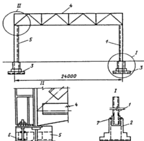
Рис. 4. Молниезащита здания II категории с металлическими фермами (в качестве токоотводов и заземлителей использована арматура железобетонных колонн и фундаментов):
