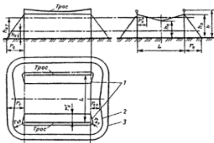
Рис. ПЗ.6. Зона защиты двойного тросового молниеотвода.
