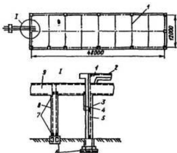
Рис 3. Молниезащита здания II категории сеткой, уложенной на кровлю под изоляцию:
