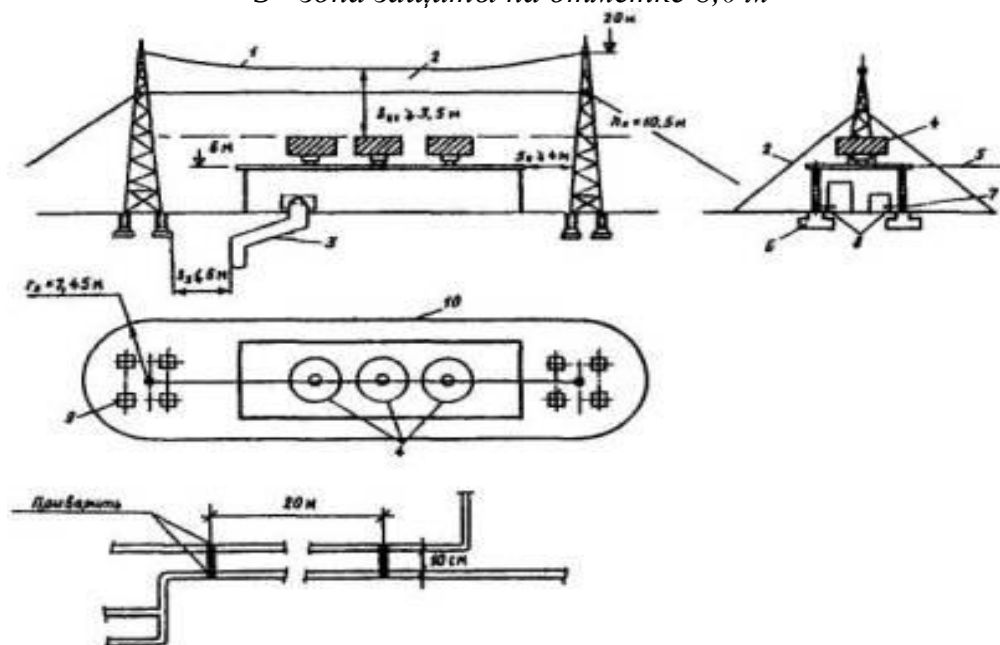
Рис. 2. Молниезащита здания I категории отдельно стоящим тросовым молниеотводом ( \rho = 300 \text{ Ом}\cdot\text{м} , S_0 \leq 4 \text{ м} , S_3 \leq 6 \text{ м} , S_{B1} \geq 3,5 \text{ м} ): 1 - трос; 2 - граница зоны защиты; 3 - ввод подземного трубопровода; 4 - граница распространения взрывоопасной концентрации; 5 - соединения арматуры, выполняемые сваркой; 6 - железобетонный фундамент; 7 - закладные элементы для присоединения оборудования; 8 - заземляющий проводник из стали 4-40 мм; 9 - заземлители - железобетонные подножки; 10 - граница зоны защиты на отметке 10,8 м
