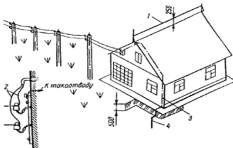
Рис. 8. Молниезащита сельского дома тросовым молниеотводом, установленным на крыше:
