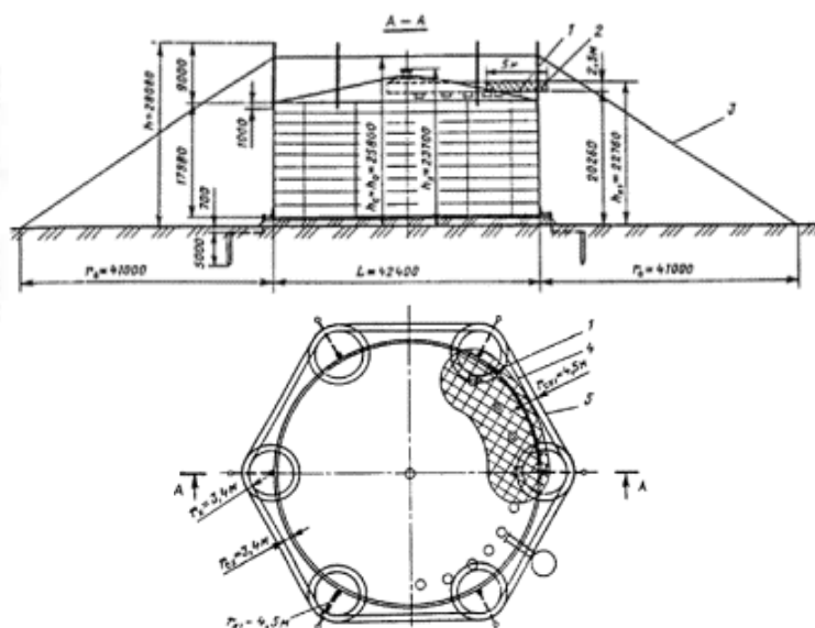
Рис. 6. Молниезащита металлического резервуара вместимостью 20 тыс. м 3 со сферической крышей:
