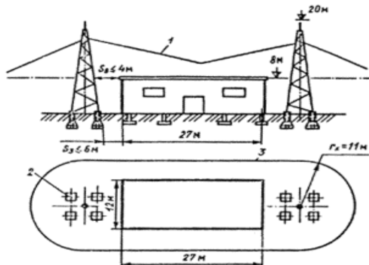
Рис. 1. Молниезащита здания I категории отдельно стоящим двойным стержневым молниеотводом ( \rho = 300 \text{ Ом}\cdot\text{м} , S_0 \leq 4 \text{ м} , S_3 \leq 6 \text{ м} ): 1 - граница зоны защиты; 2 - заземлители-подножки фундамента; 3 - зона защиты на отметке 8,0 м
